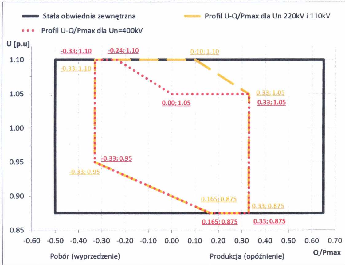
Profil U-Q/Pmax modułu parku energii
